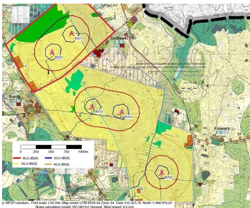
Rys. 7. Pole akustyczne projektowanej farmy elektrowni wiatrowych z wyszczególnieniem przedmiotowego obszaru opracowania (linia koloru czerwonego).
