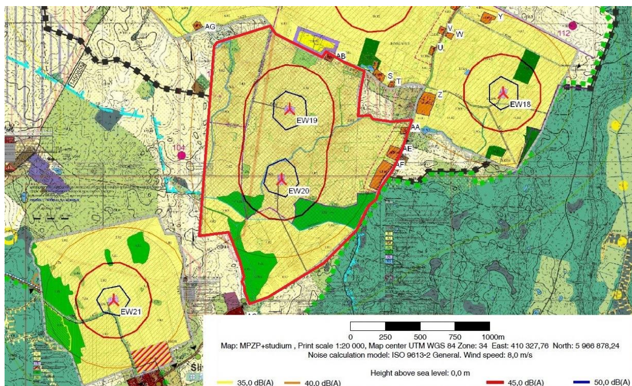
Rys. 7. Pole akustyczne projektowanej farmy elektrowni wiatrowych z wyszczególnieniem przedmiotowego obszaru opracowania (linia koloru czerwonego).
