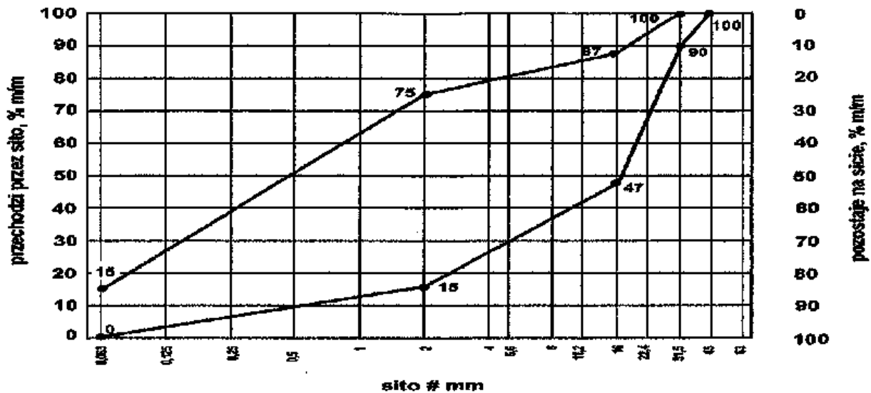
Rys. 1. Krzywe graniczne uziarnienia mieszanki kruszyw 0/31,5 mm do górnej warstwy podłoża ulepszonego Tablica 3. Wymagania wobec mieszanek kruszywa niezwiązane w warstwie podłoża ulepszonego Skróty użyte w tabelicy: Kat.–kategoria właściwości, wsk.– wskaźnik, wsp. – współczynnik
